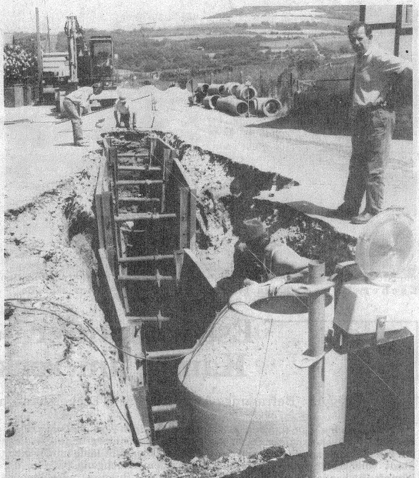
Reileifzen. Die Abwasserbeseitigungs-Aufgaben der Kommunen hat den Gemeinden des Kreises Holzminden in den letzten Jahren manche „Großbaustelle“ beschert. Jetzt ist Reileifzen an der Reihe mit dem Bau des Kanalnetzes
